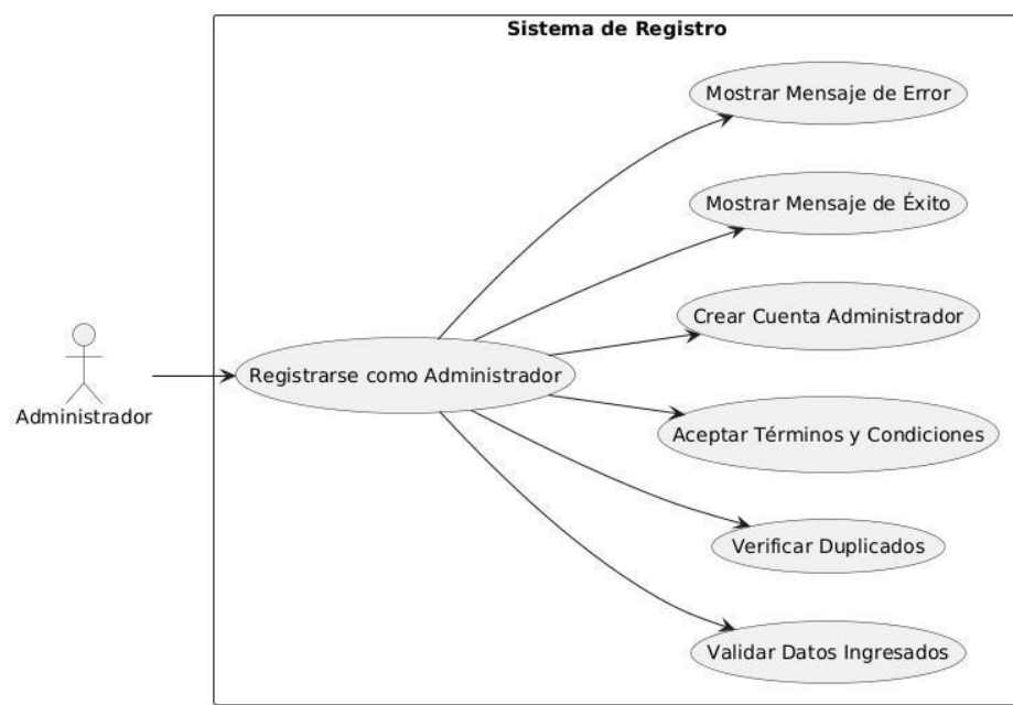
Diagrama de Caso De Uso CU-01
